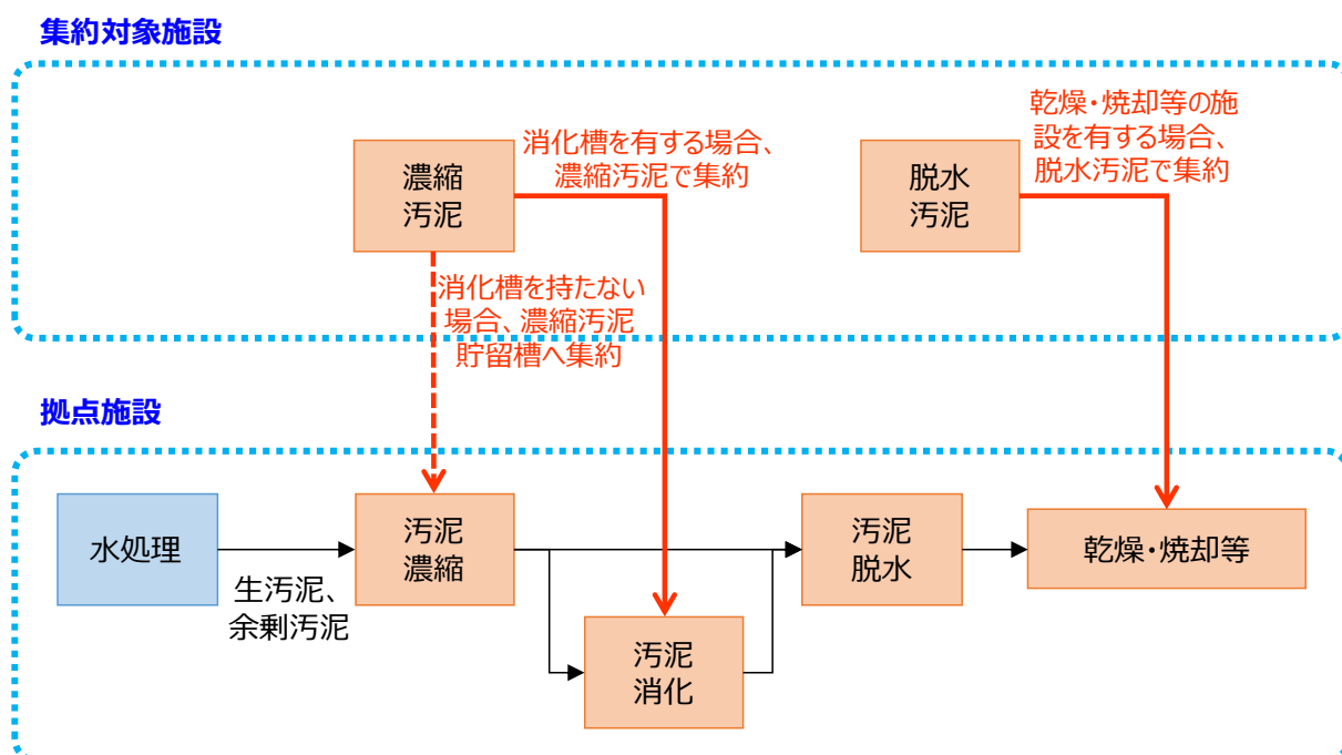
図 3.5 拠点施設で集約可能な主な汚泥形態の条件設定
