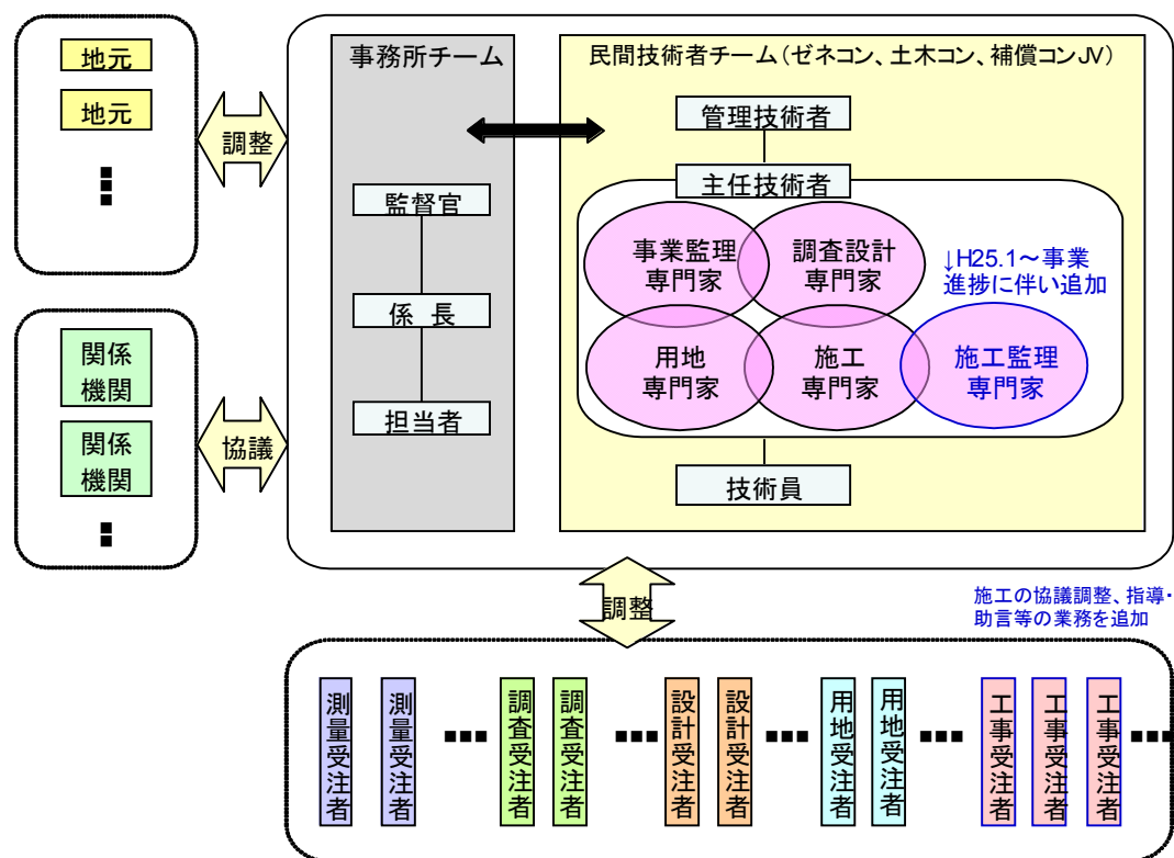
図 3-6 事業促進 PPP の実施体制 6
