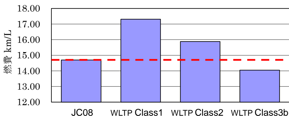
図2 Class2 が適用される車両(最高速度 120km/h 以上)における各サイクル(超高速フェーズは除外)での燃費試験の結果
