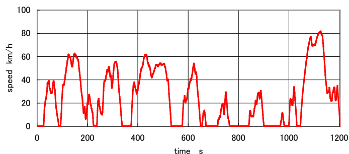
図1 乗用自動車及び貨物自動車(車両総重量 3.5t 以下)の燃費測定方法の走行モード(JC08 モード)
