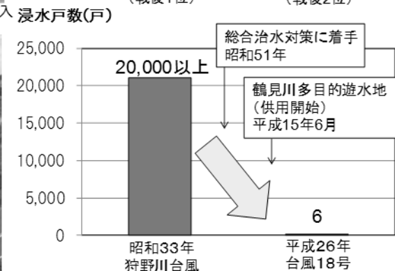
平成26年台風18号では、戦後2番目の雨量を記録したものの、浸水戸数は6戸
