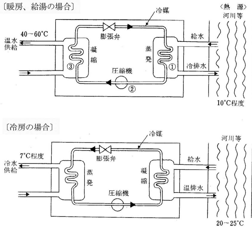
図 ヒートポンプによる熱利用の例
