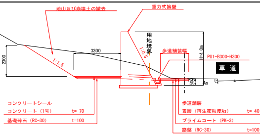
【断面図(A-A断面)】
