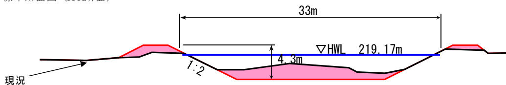
標準断面図 (A-A断面)
