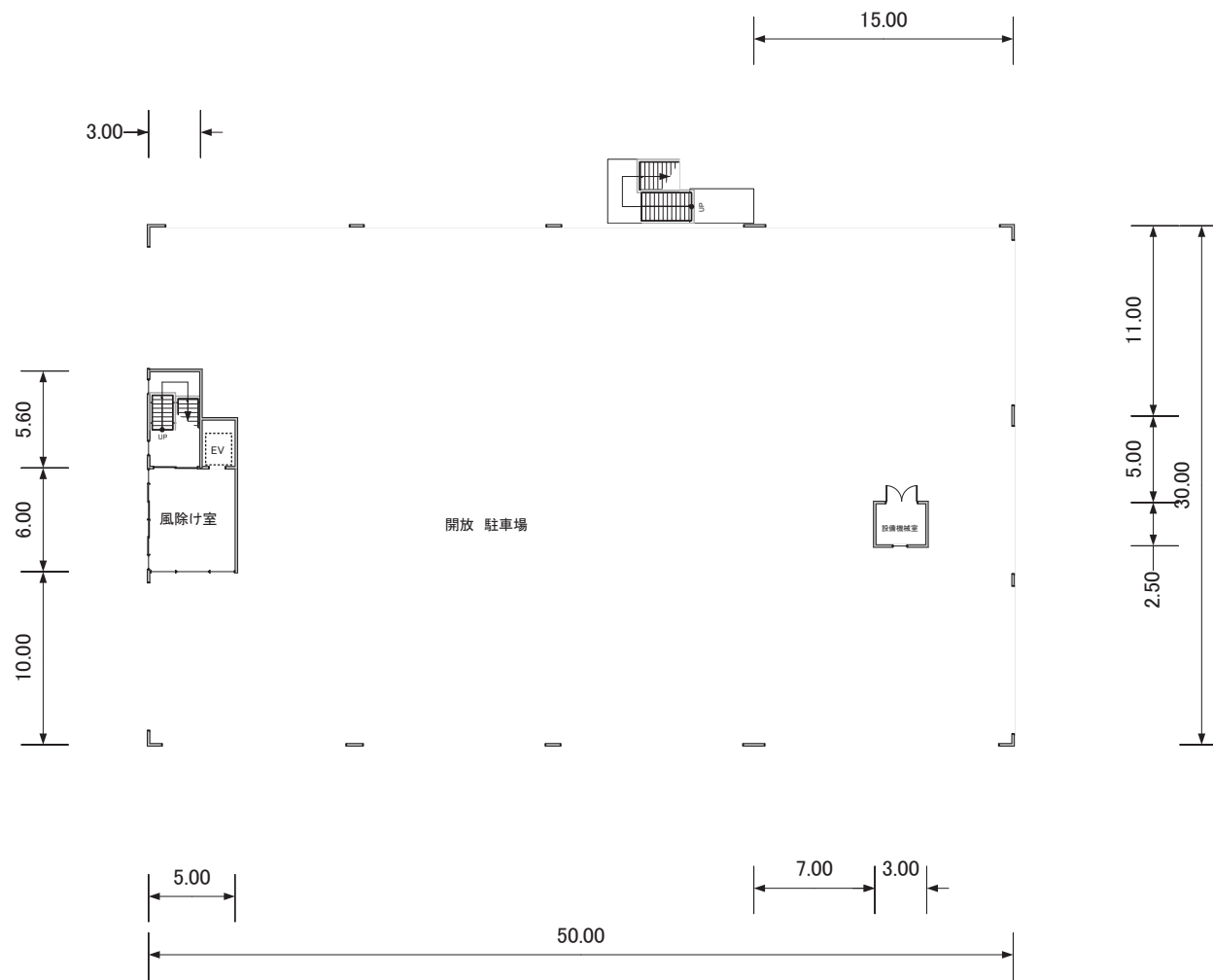
飲食店 1F平面図
