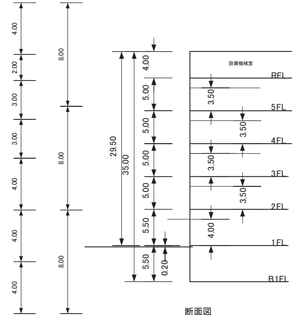
断面図
