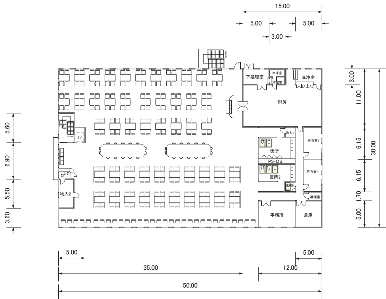
飲食店 2F平面図
