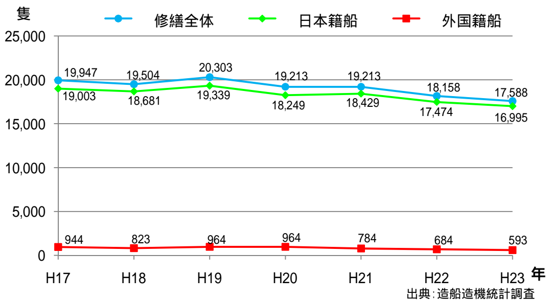
修繕実績（隻数）の推移
