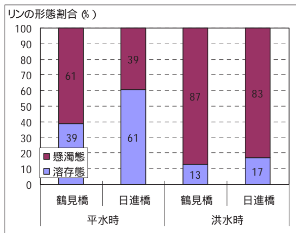
図 4-20 平時・洪水時の流出負荷量と形態の割合
