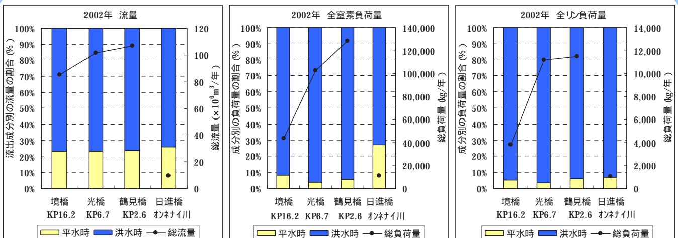
図 4-19 平時・洪水時の流出負荷量とその割合
