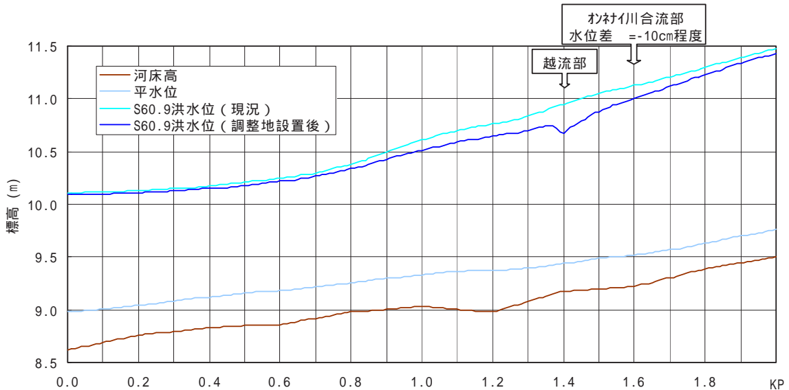
図 4-21 土砂調整地による洪水位低減効果
