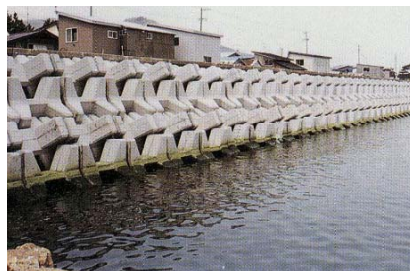
消波堤
