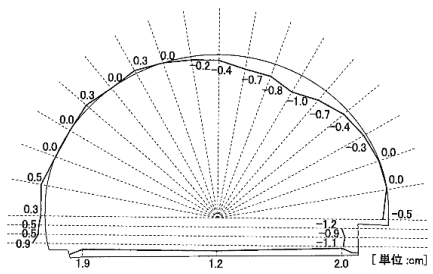
断面計測結果のとりまとめ
