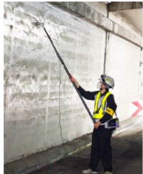
点検者から離れた位置を打撃し、打撃波形から打音異常を判定
