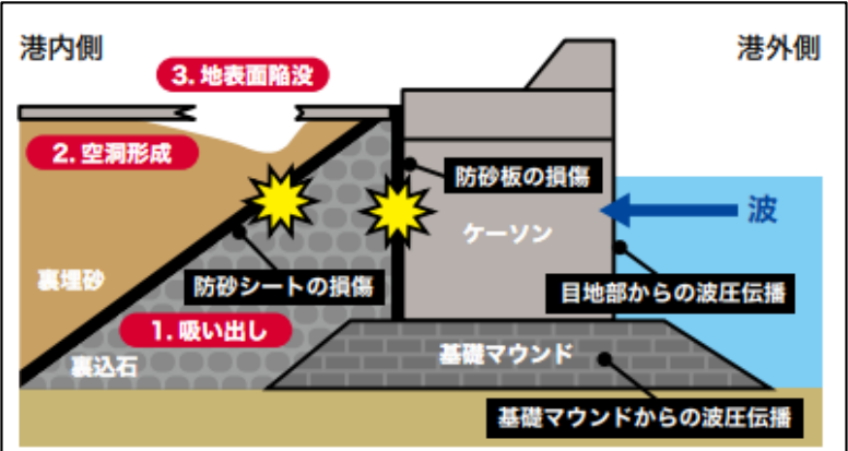
ケーソン護岸における吸い出しの概念図
