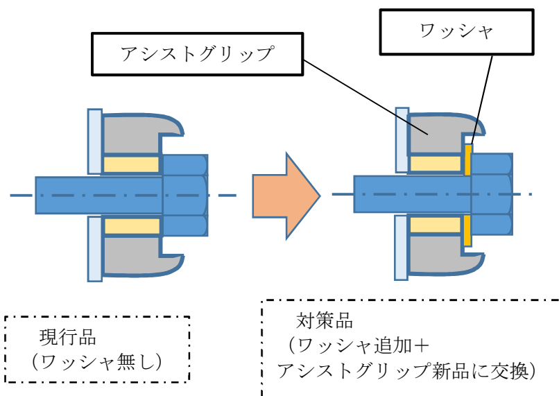
助手席アシストグリップ組み付け部
