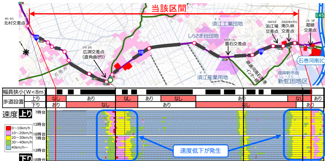
図3 対象区間の道路状況・旅行速度 資料：MICHIデータ・ETC2.0プローブ情報(H31.4～R1.6 平日)
