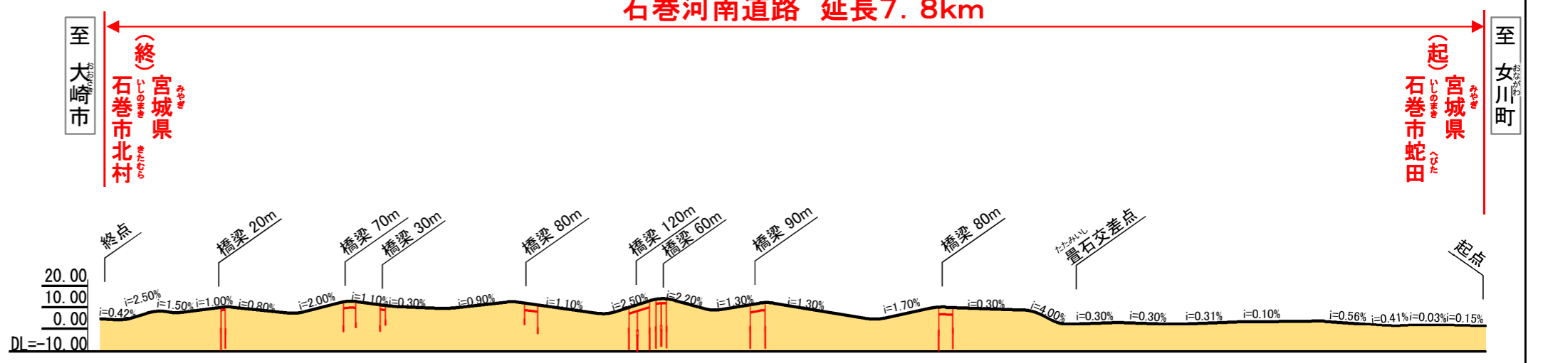
計画縦断図
