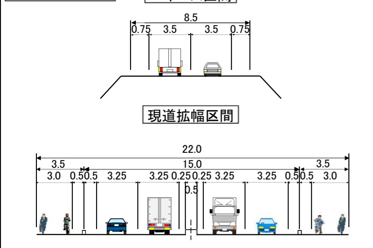
標準横断図 [m]
