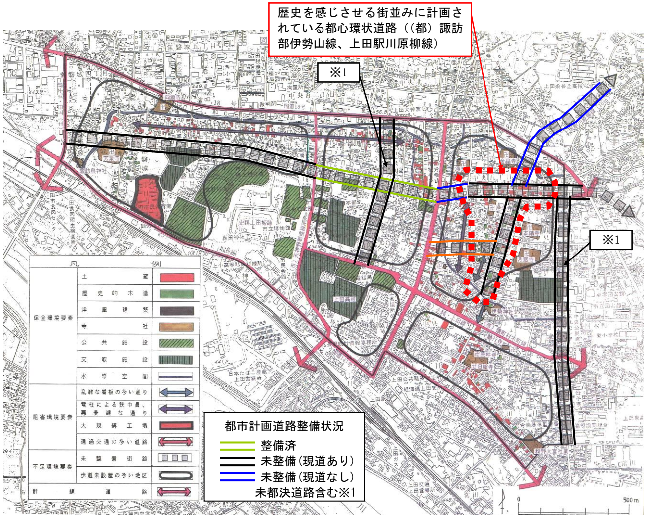
図 2-56 地区整備に向けた課題図（保全環境要素と阻害要素）
