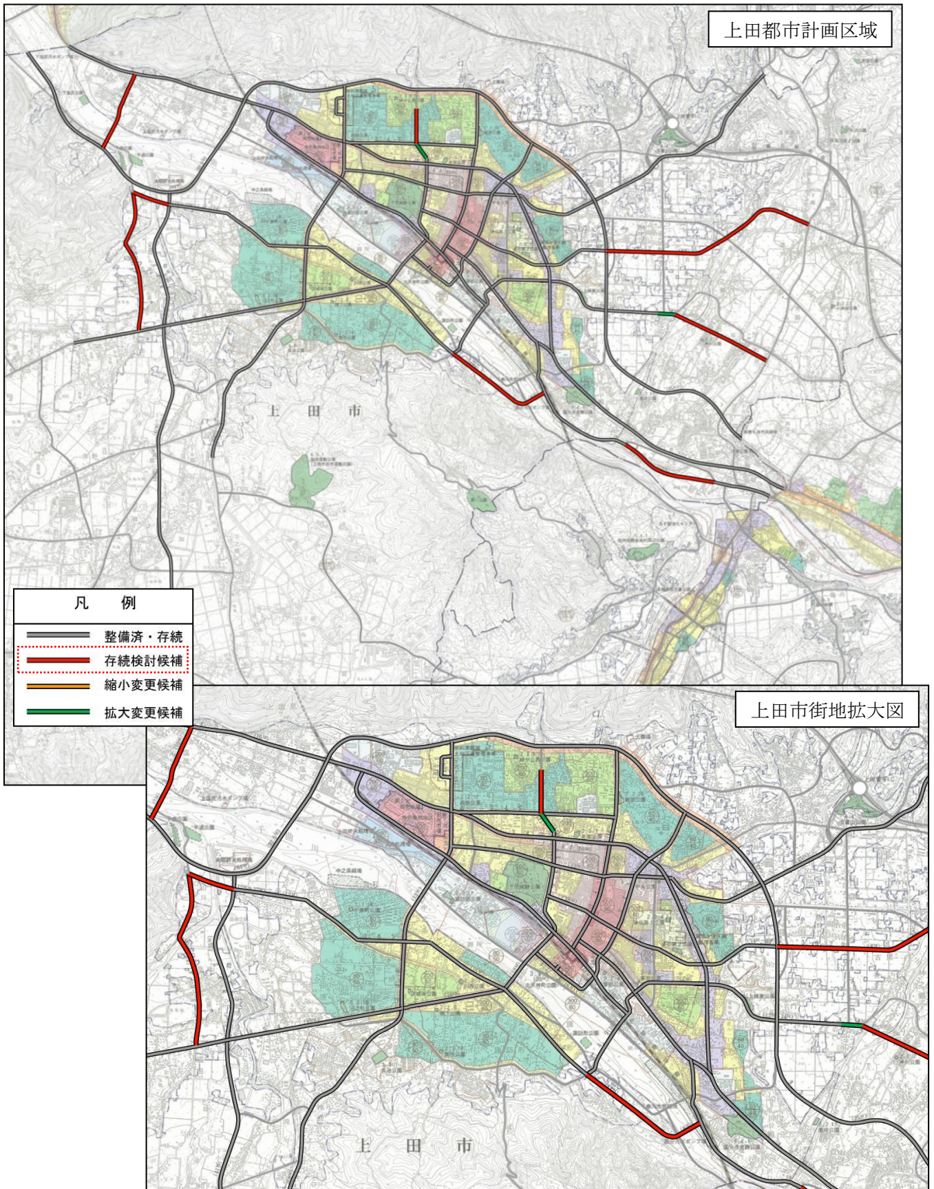
図 2-51 都市計画道路見直し案
