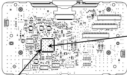
マルチインフォメーションディスプレイ裏面
