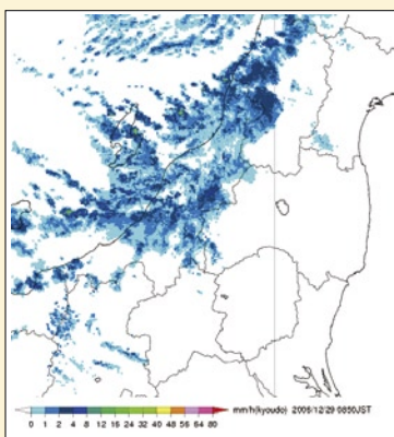
冬の雷の気象レーダー画像 (2006年12月29日) 雪雲が新潟県を覆っています。夏ほど発達はしていませんが、日本海側に雷をもたらします。
