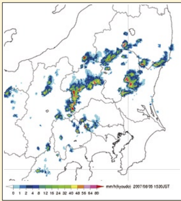
夕立の気象レーダー画像 (2007年8月5日) 群馬県や栃木県を中心に雨雲が点在しています。 青→緑→黄→赤となるにつれて雨雲が発達していることを表しています。
