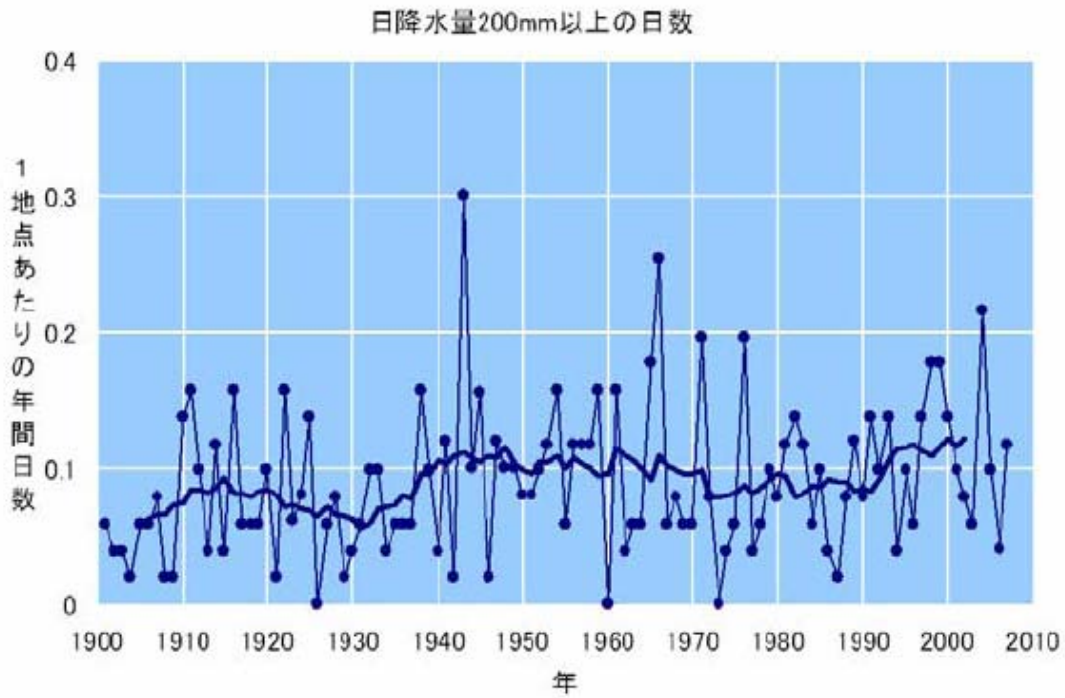
図1 全国51地点の観測値から得られた日降水量200ミリ以上の年間発生日数の長期変化。年々の値（細線）と11年移動平均値（太線）を示す。
