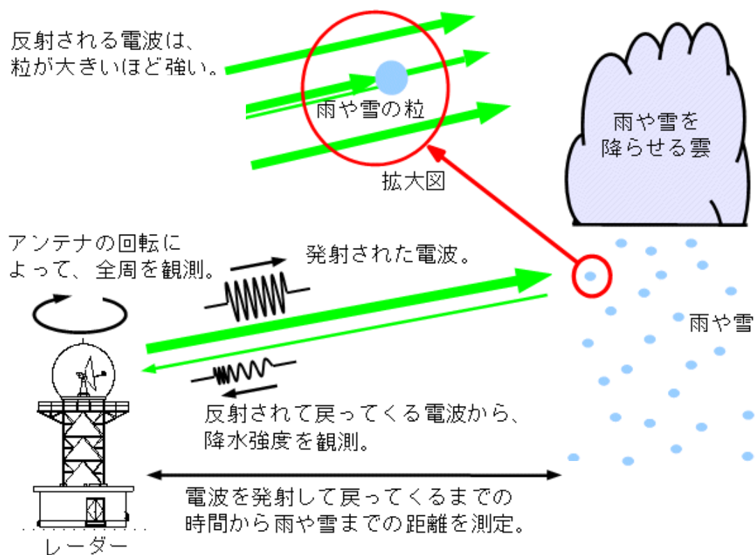
《気象レーダーの観測原理》
